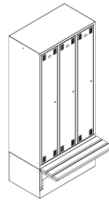
G13UB UB SB 1 Abteil vertikal 3 Abteil horizontal
