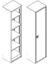
U500 4 verstellbare Tablare Türe einflügelig rechts oder links
