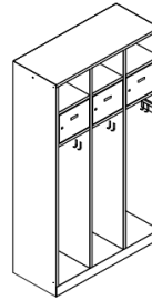
FW32 1 Kleiderabteil vertikal 3 Abteil horizontal Schliessfach Helmfach
